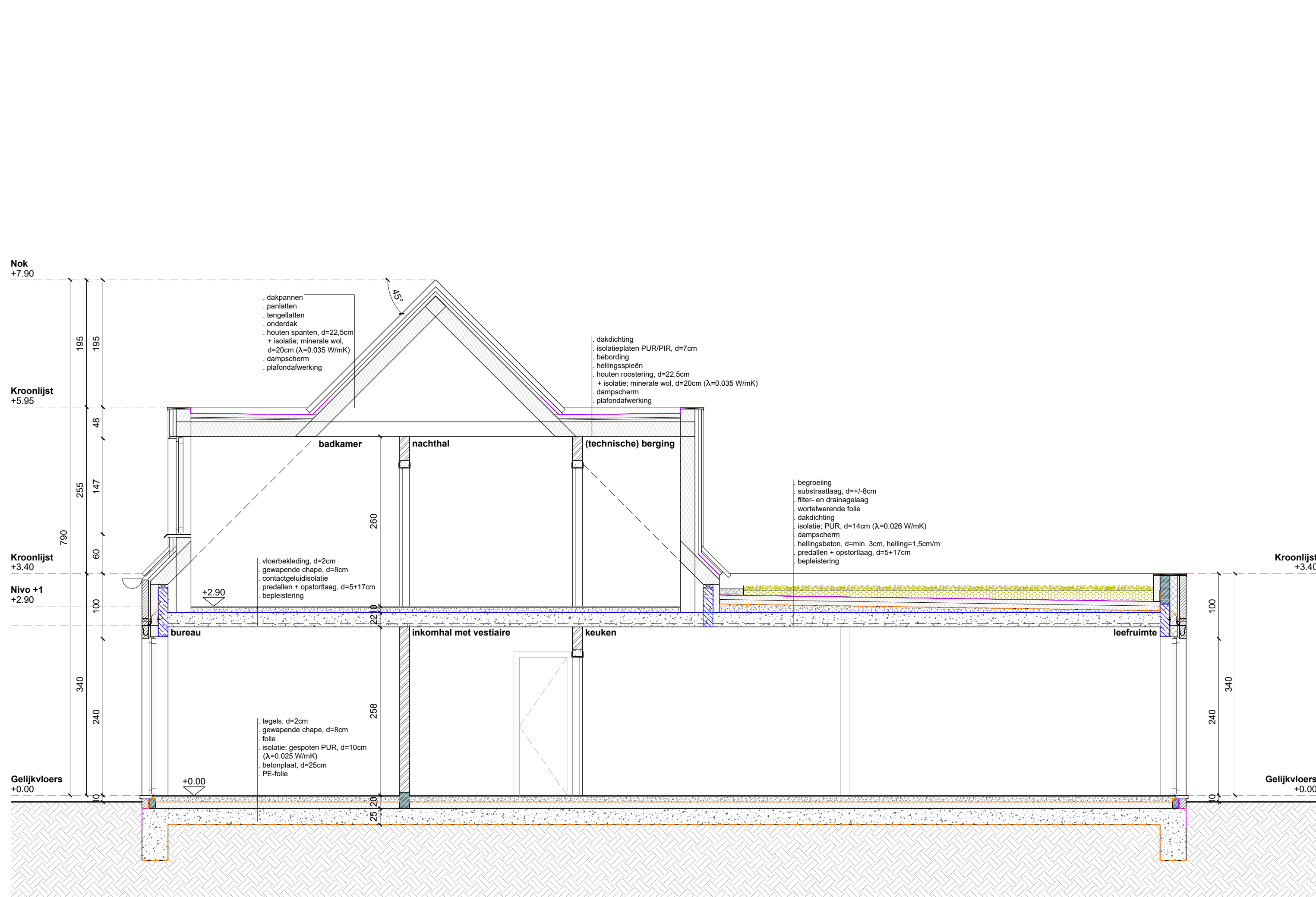
SNEDE
