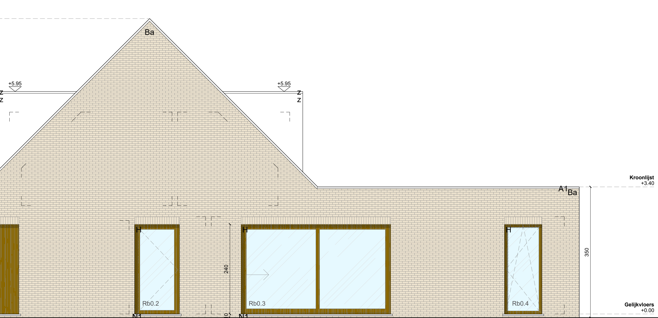
ZIJGEVEL RECHTS
