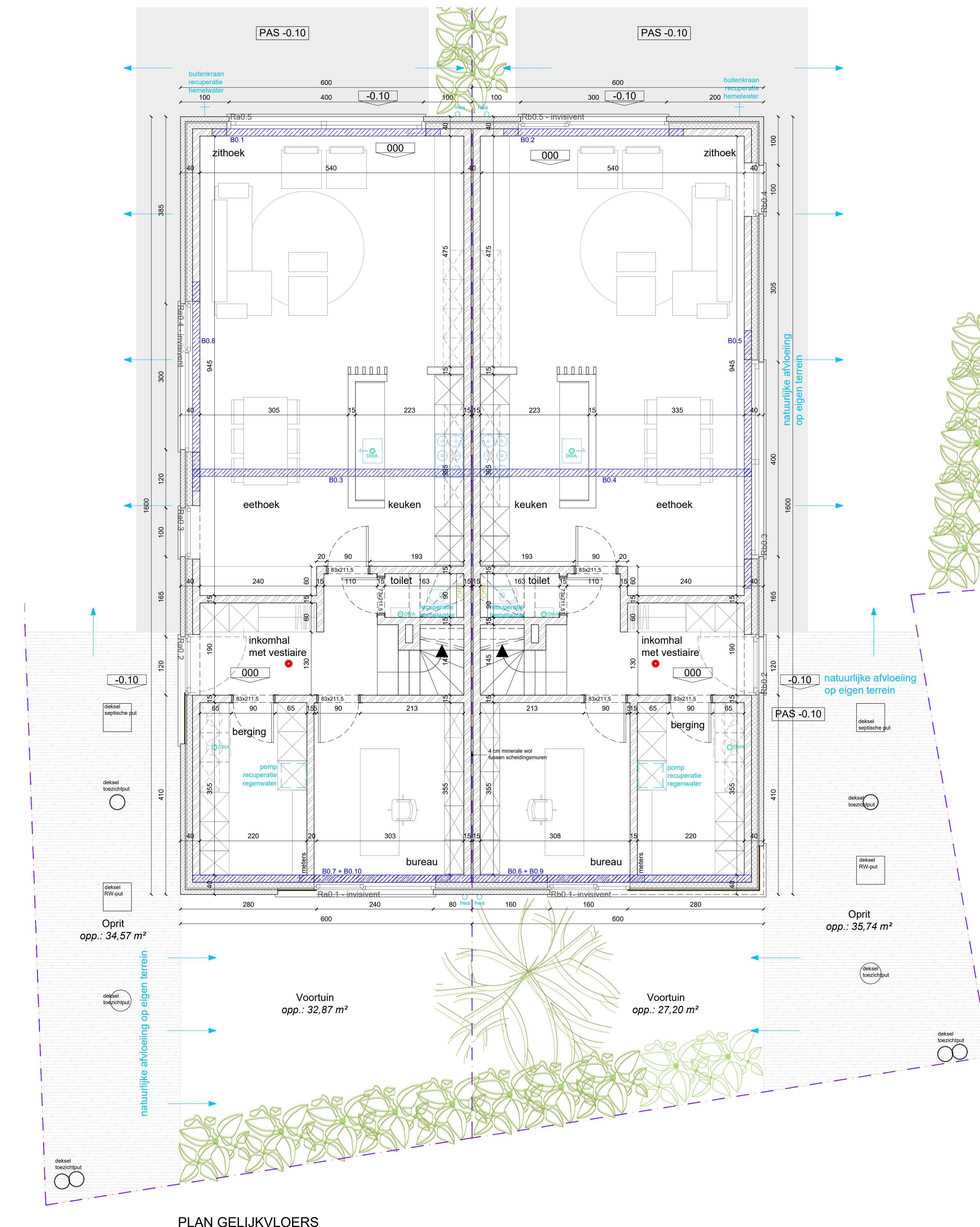
PLAN GELIJKVLOERS
