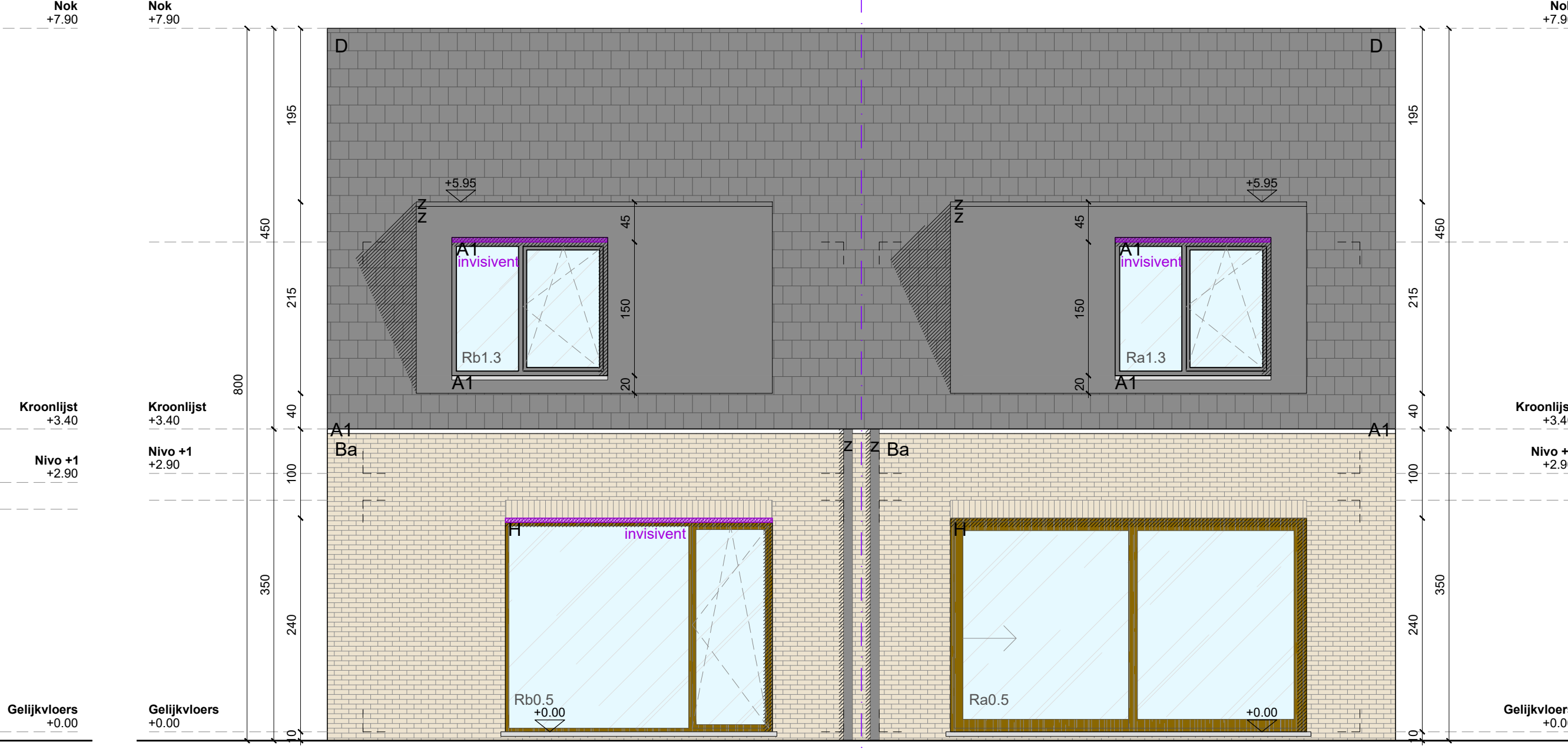
ACHTERGEVEL
